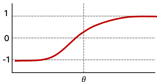
【 Tanh 】
