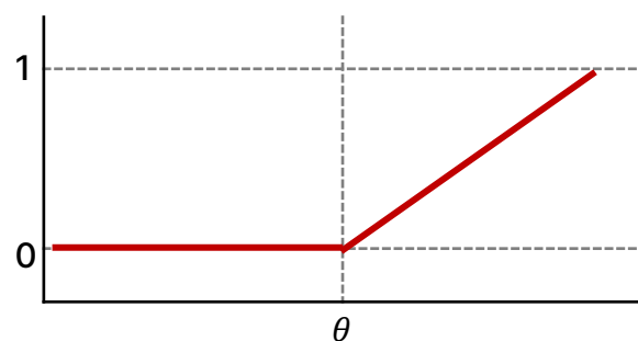
【 ReLU 】
