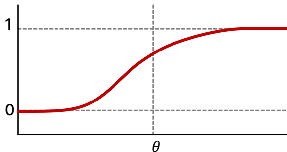
【 Sigmoid 】
